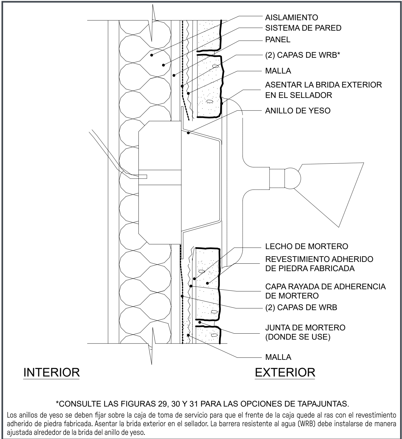
Figura 31. Penetración, accesorio
